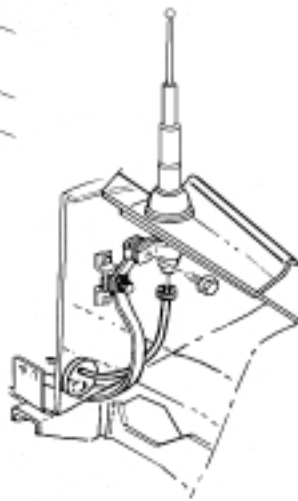
1 - Antenna
